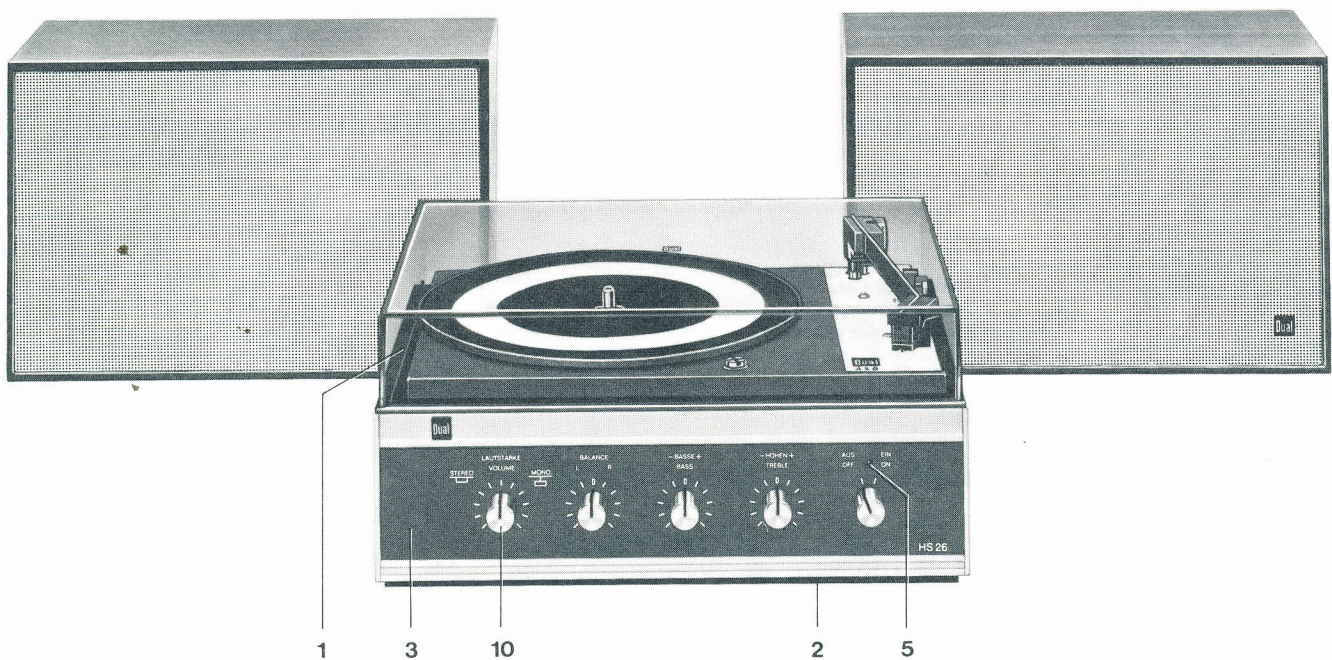
Fig. 5 Stereo-Heimanlage Dual HS 26
