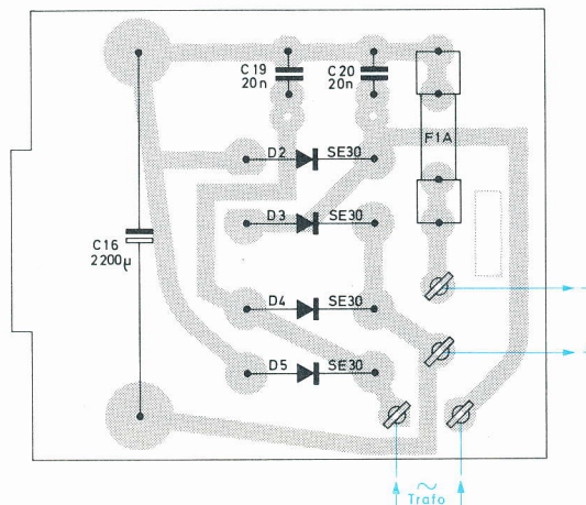
Fig. 4 Ätzsaltplatte der Stromversorgung 222 747 (Leiterseite)
