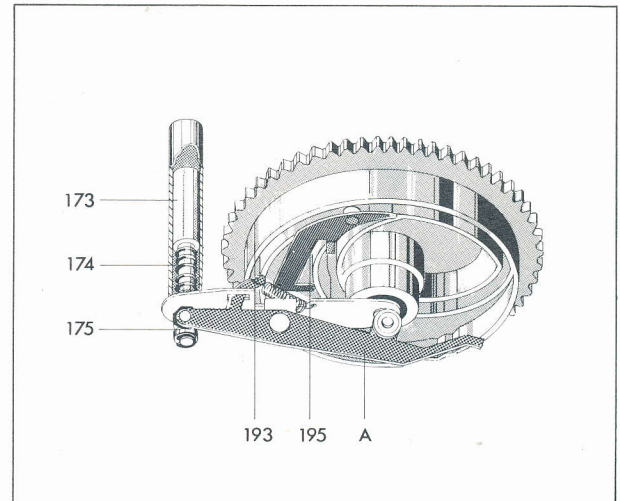
Fig. 16 Wechselvorgang
