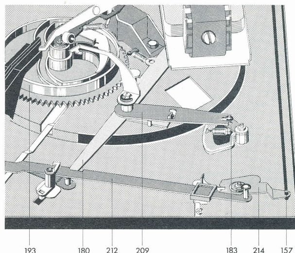
Fig. 12 Stoppstellung
