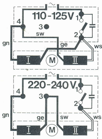
Fig. 5 Anschluß der Feld- spulen (ohne Anschlußplatte)
