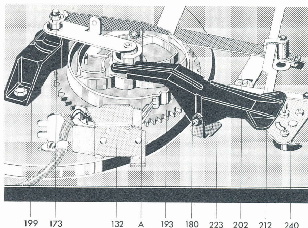
Fig. 9 Kinematik der Tonarmsteuerung
