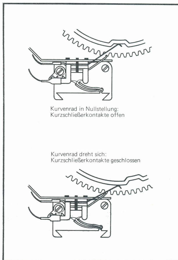
Fig. 13 Kurzschließer
