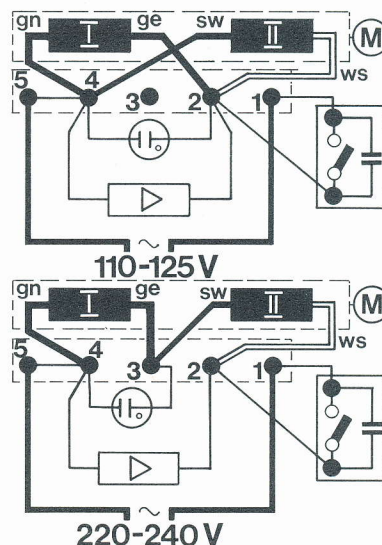
Fig. 6 Anschluß der Feld- spulen (mit Anschlußplatte)
