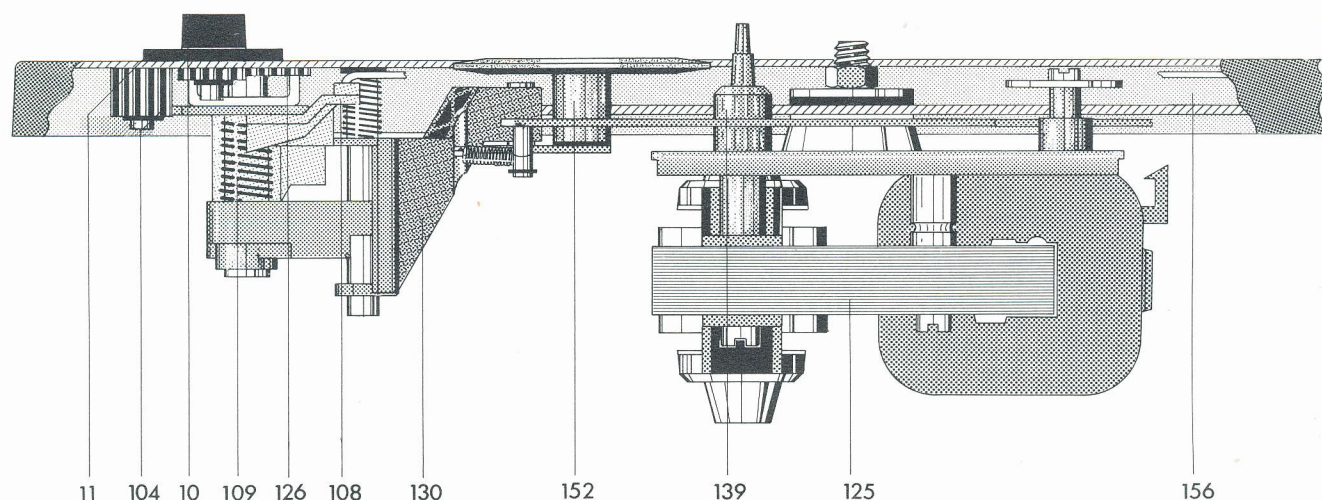
Fig. 2 Motoraufhängung und Antrieb des Plattentellers Dual 1220
