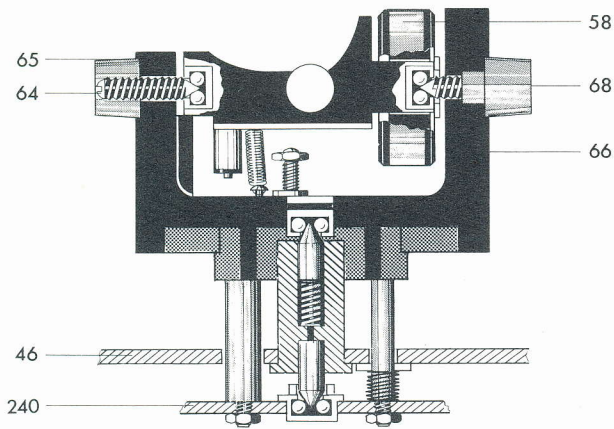
Fig. 7 Tonarmlagerung
