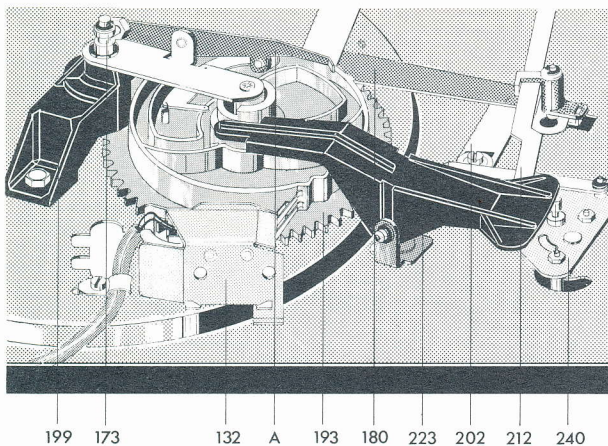
Fig. 14 Schallplattenabwurf
