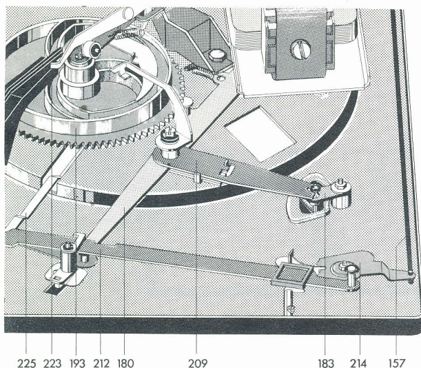
Fig. 11 Startstellung
