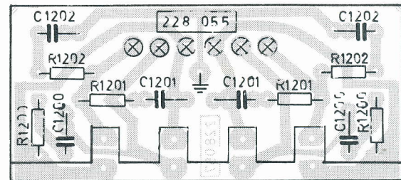
Lautsprecheranschlußplatte Speaker connection board Plaque de connection de haute-parleur
