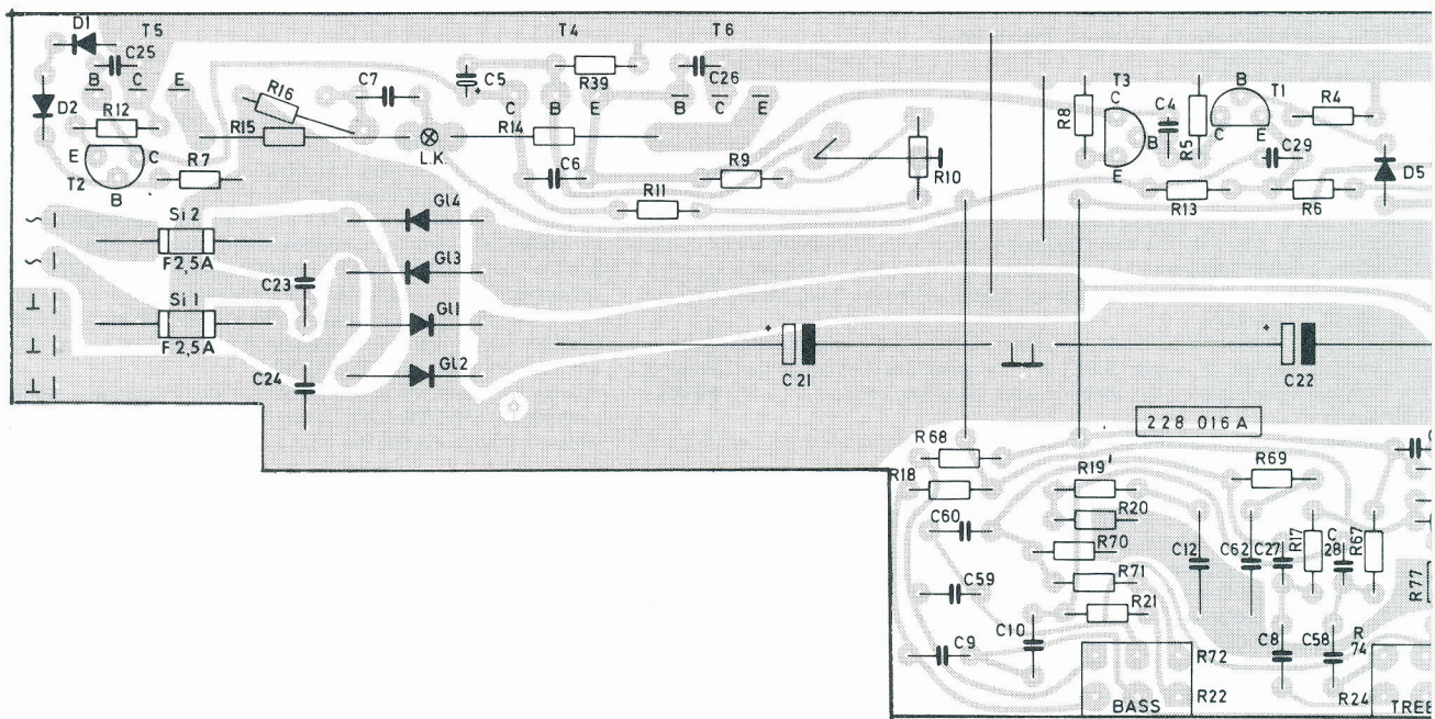
Verstärkerplatte Amplifier board Etag amplificateur
