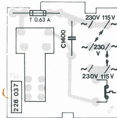
Netzplatte Power board Plaque secteur
