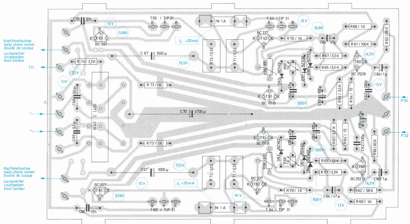
Fig. 5 Ätزشaltplatte des Endverstärkers 227 587 (Leiterseite)
