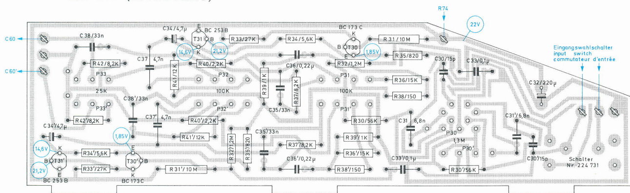
Fig. 4 Ätزشaltplatte des Regelverstärkers 227 586 (Leiterseite)
