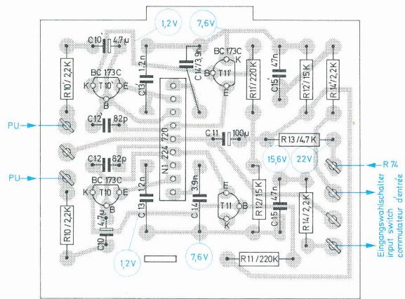
Fig. 2 Ätزشaltplatte des Vorverstärkers 227 585 (Leiterseite)
