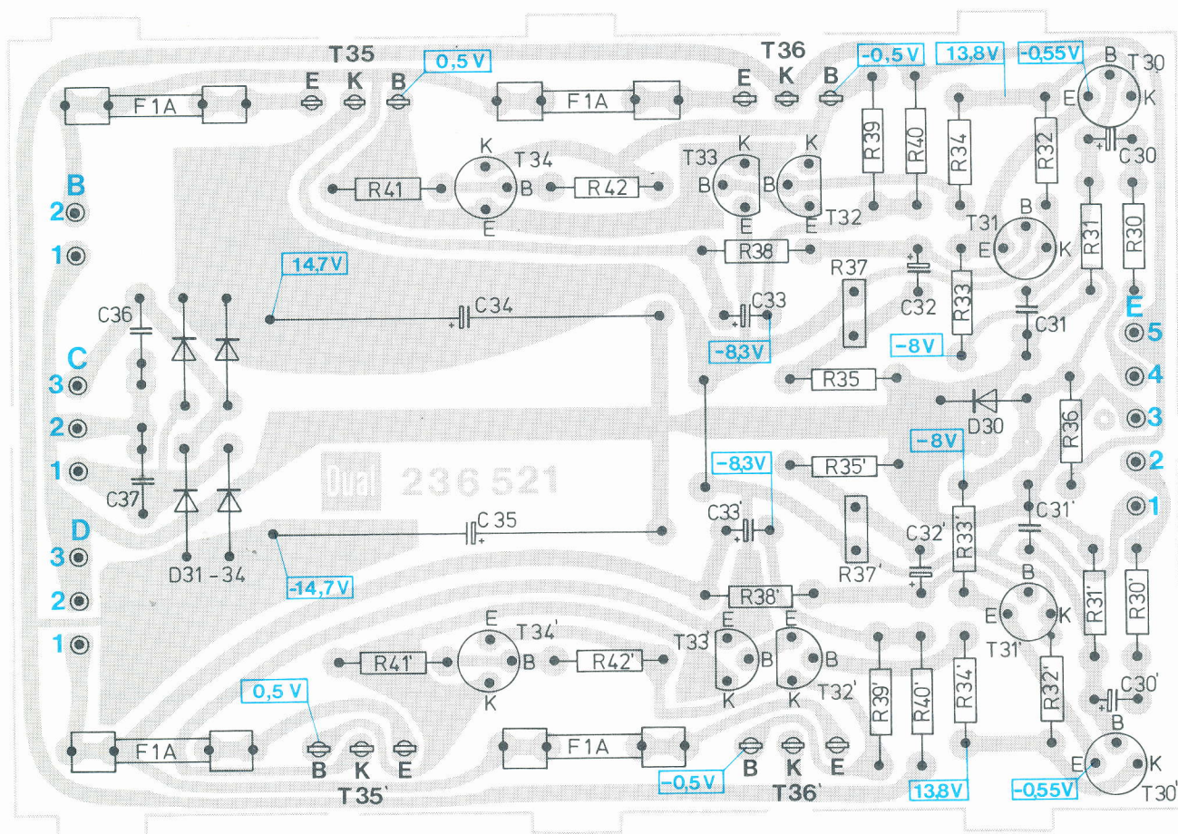
Fig. 3 Endverstärker 239 598 (Leiterseite)
