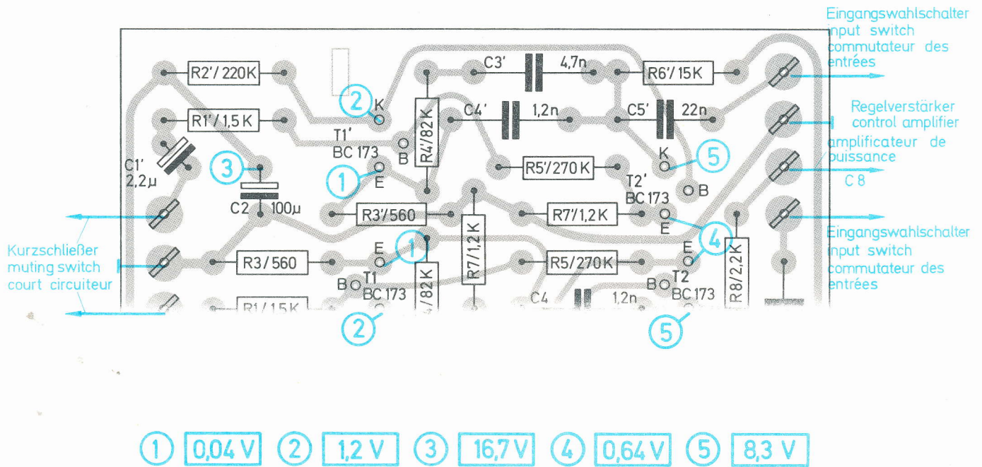
Fig. 7 Ätzschatplatte des Vorverstärkers 217 650 (Bestückungsseite)
