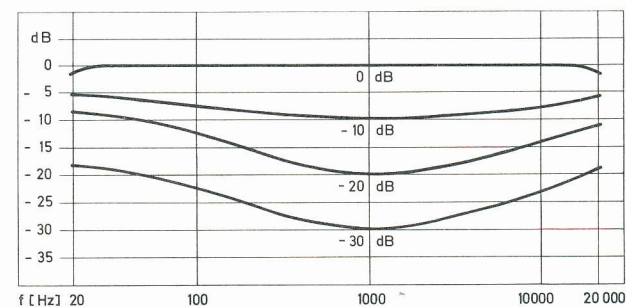
Fig. 5 Wirkungsweise der physiologischen Lautstärkeregelung 0 dB = Lautstärkeregelner offen
