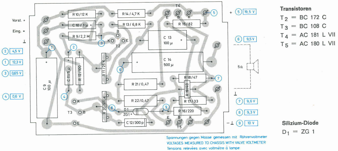
Fig. 7 Ätzschnplatte Endstufen-Einheit 36 W - U 10 (Bestückungsseite)
