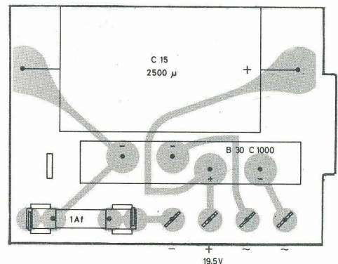
Fig. 1 Ätzschriftplatte für Netzteil 36 W - U 4
