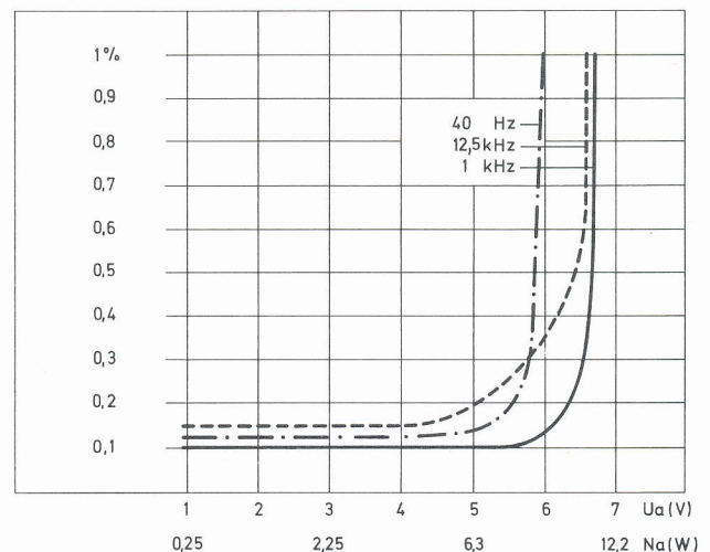
Fig. 3 Klirrgrad bei 40 Hz, 1000 Hz, 12 500 Hz in Abhängigkeit von der Ausgangsleistung
