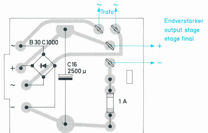
Fig. 2 Ätزشaltplatte 213 869 für Netzteil (Leiterseite)
